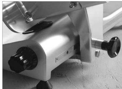
Schlittenfixierung
